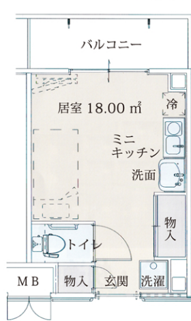
■間取図
